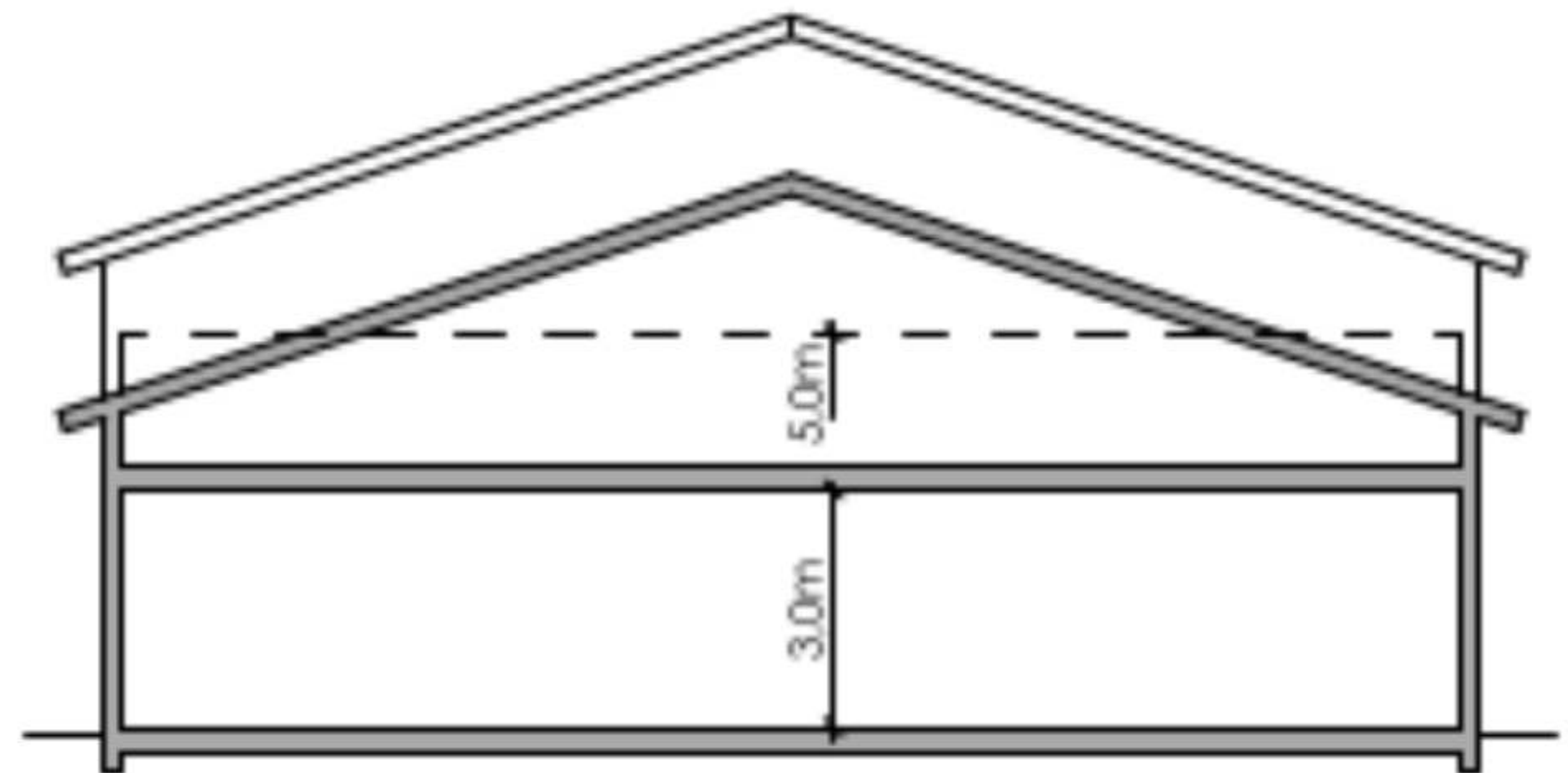
LEIKKAUS A-A
